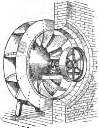
FIG. 33.—Cone fan inlet side.
